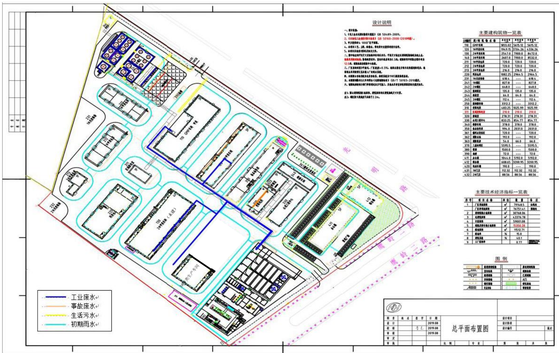
附图4 项目厂区雨污管网图
