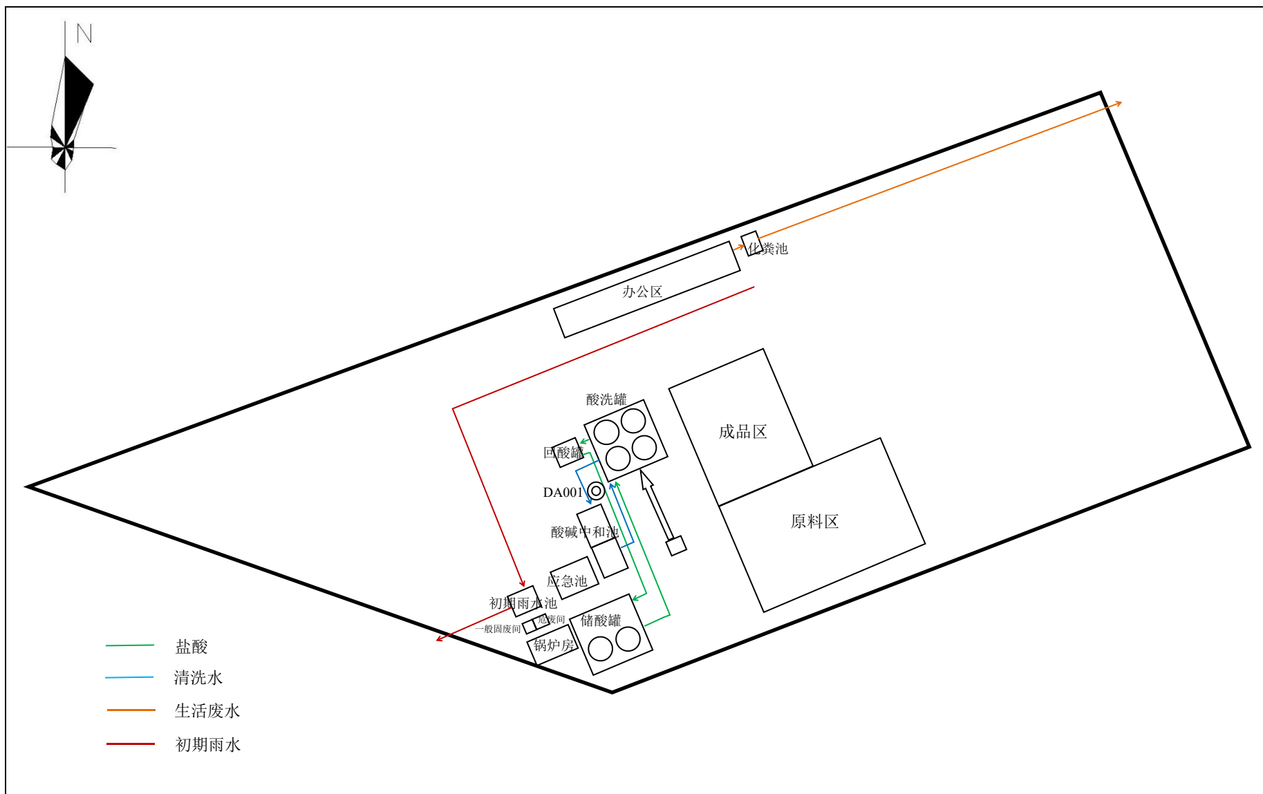
附图5 项目雨污管网图
